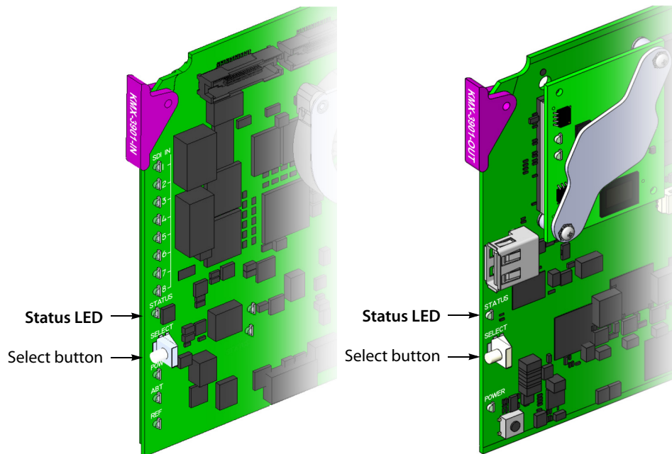
Front edge of a Kaleido-MX 4K input card
