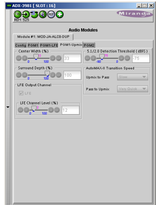
Figure 6.22 JA-ALC module - Upmix
