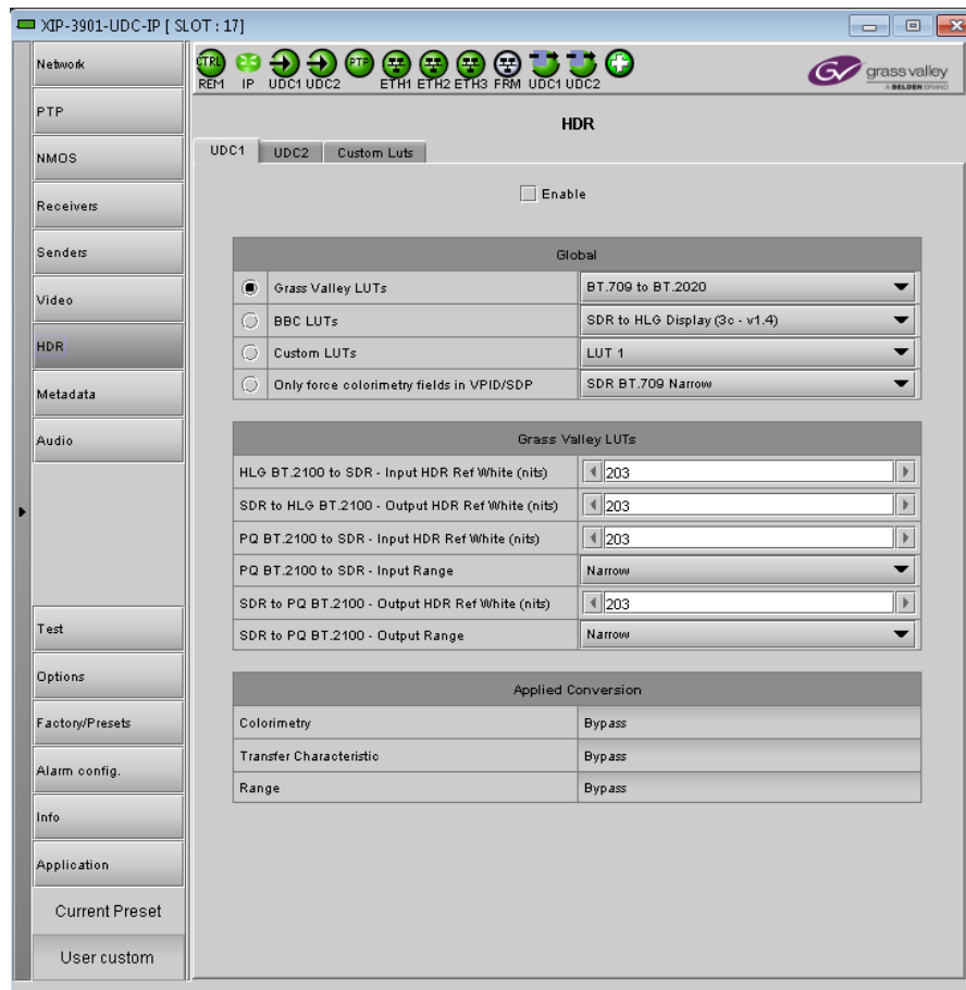
Figure 69 – HDR UDC1 / UDC2 Tab
